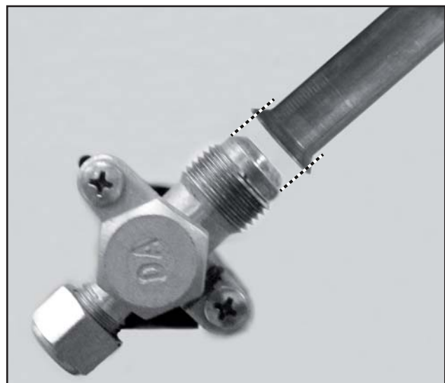
FIGURA 22 - CONEXÃO NIPLE TUBO
