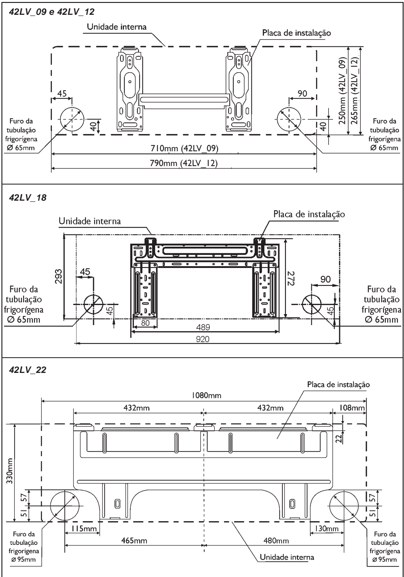
FIGURA 13 - SUPORTE DE MONTAGEM E DIMENSÕES
