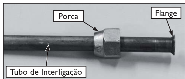
FIGURA 21 - TUBO COM PORCA
