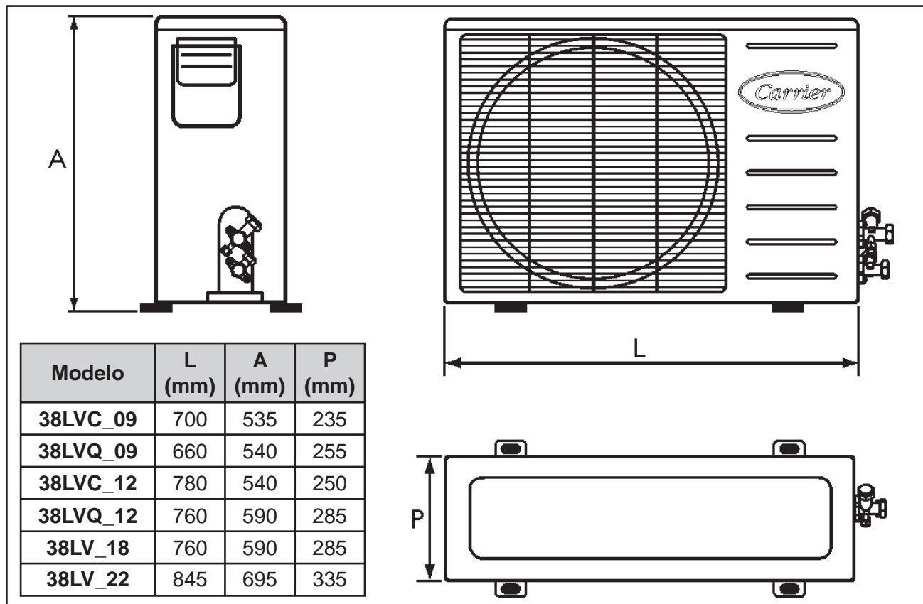
FIGURA 2 - DIMENSIONAMENTO
