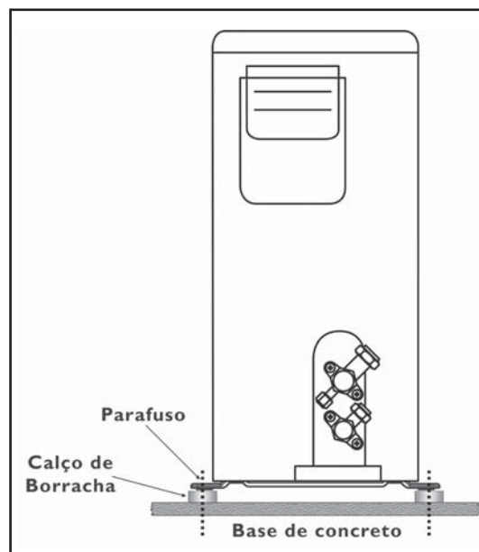
FIG. 4 - INST. SOBRE BASE NO PISO
